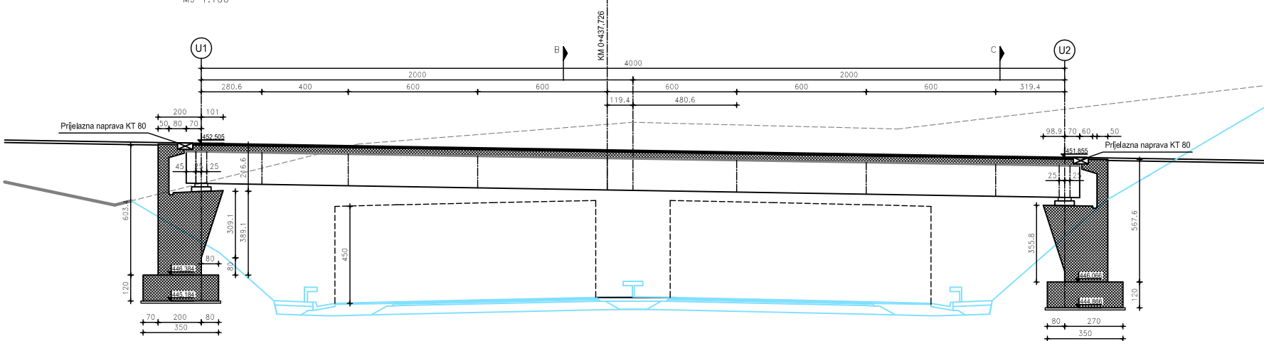
UZDUŽNI PRESJEK U OSI NOSAČA MJ 1:100
