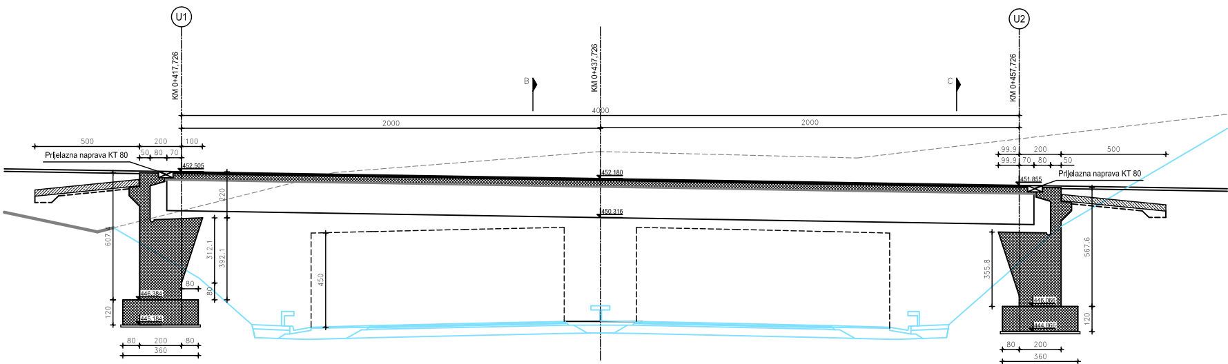
UZDUŽNI PRESJEK U OSI PRIJELAZA A-A MJ 1:200
